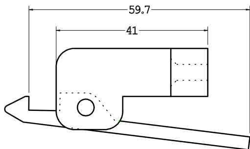
Cod. BLCAL17 Blocca cassette alluminio
